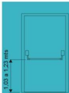
DIMENSIONES PARA LA COLOCACION PUERTA VISTA DEL LADO INTERIOR
